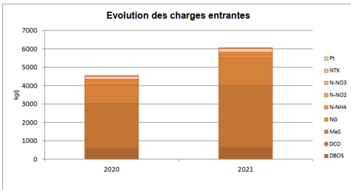
Evolution des charges entrantes au niveau de la STEP de Dreux – Rapport annuel 2021
