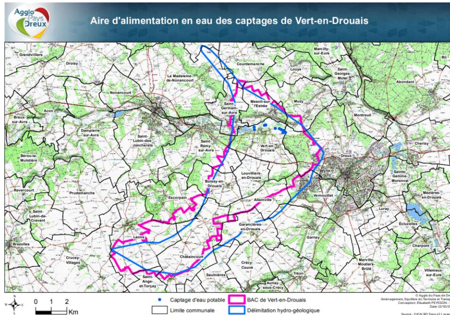
Aire d'alimentation en eau des captages de Vert-en-Drouais – SCoT du Pays de Dreux
