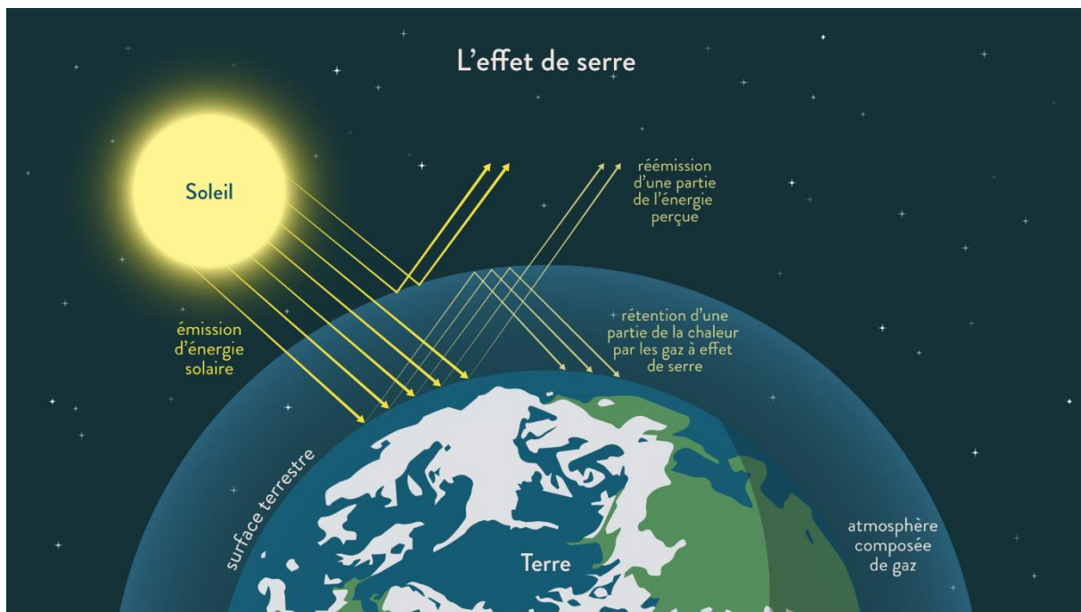
L'effet de serre. Source : Schoolmouv
