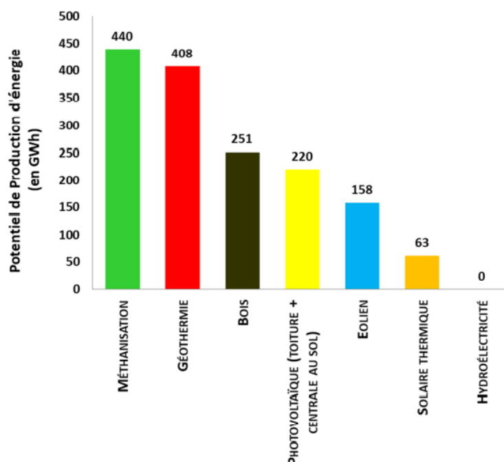
Répartition du potentiel de développement en EnR par type de production sur la CA du Pays de Dreux
