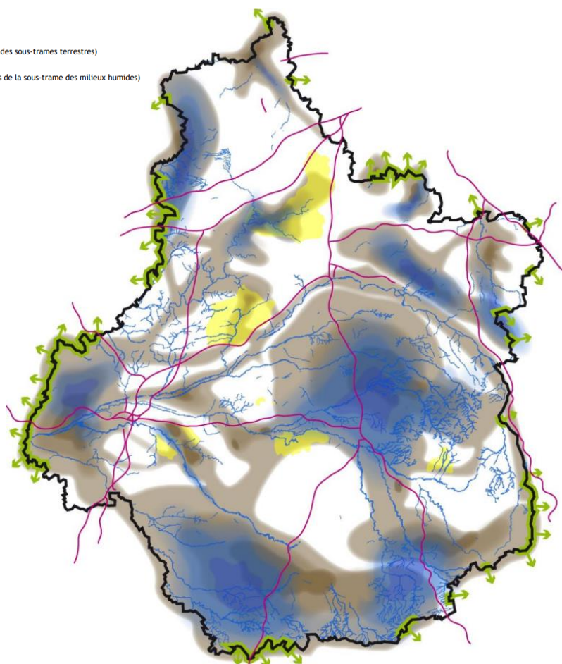
Carte schématisant de la TVB de la région Centre-Val de Loire - SRCE repris dans le SRADDET 2020
