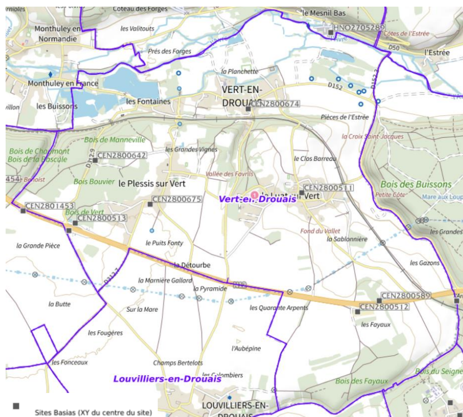
Localisation des sites BASIAS (en noir) et BASOL (en rose) sur le territoire. Source : Géorisques
